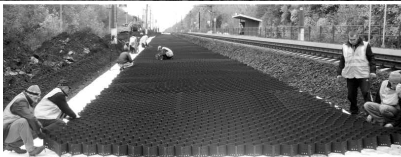
Самый современный способ укрепления балластного слоя — георешетка. Благодаря ей нагрузка на земляное полотно распределяется равномерно
